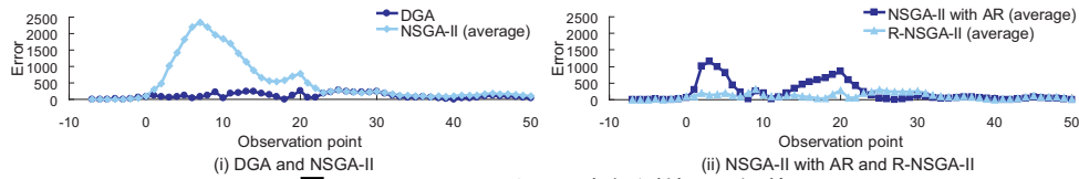
図 2: HIDECS における各観測値との誤差
